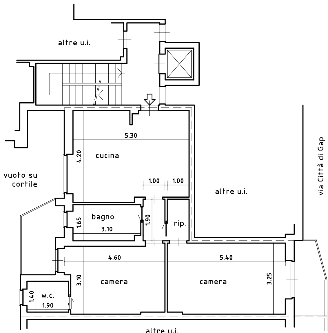
PIANO SECONDO ESISTENTE SCALA 1:100
