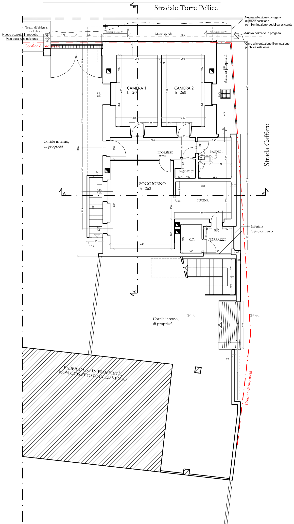
Pianimetria piano terra
